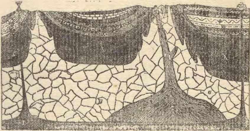
Idealer Durchschnitt eines Teiles der Erdrinde.
